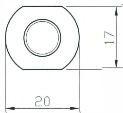
Flange
