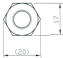
Nut
